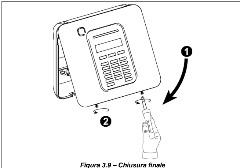
Figura 3.9 – Chiusura finale
