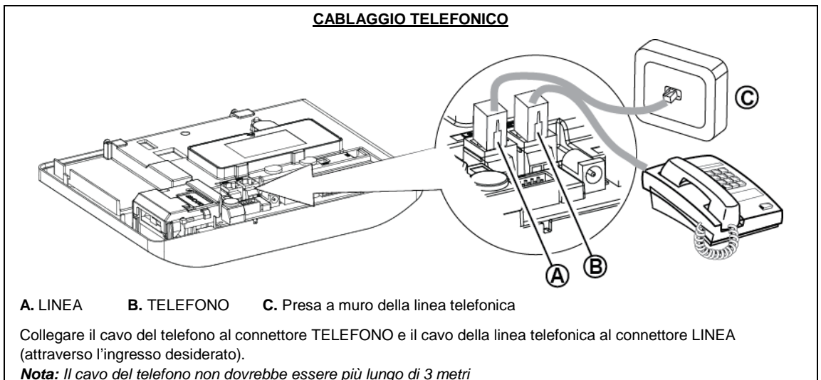
Figura 4.3a – Cablaggio telefono
