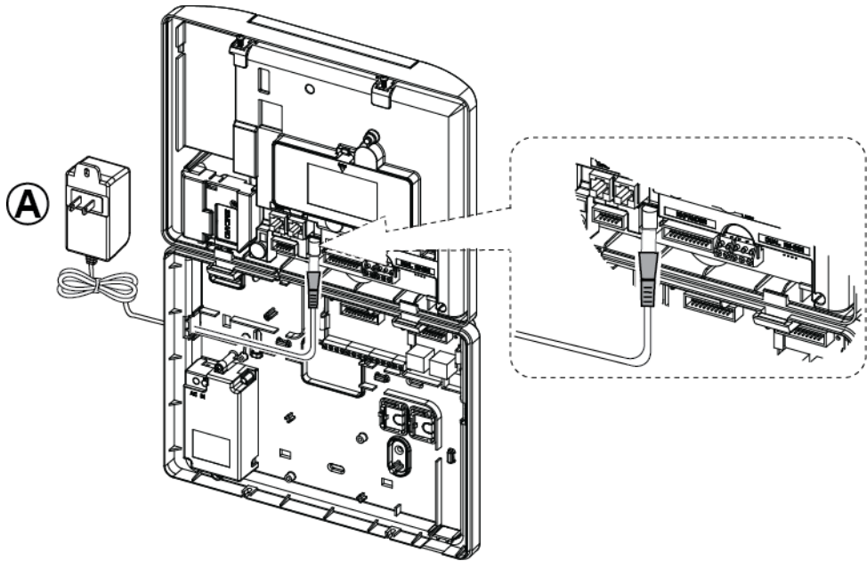
Figura 4.10b – Collegamento alimentatore esterno
