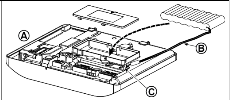
Figura 4.11 – Inserimento batterie
