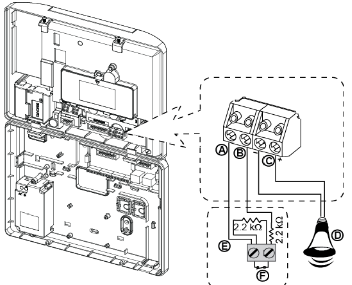
Figura 4.4 – Cablaggio zona cablata e sirena
