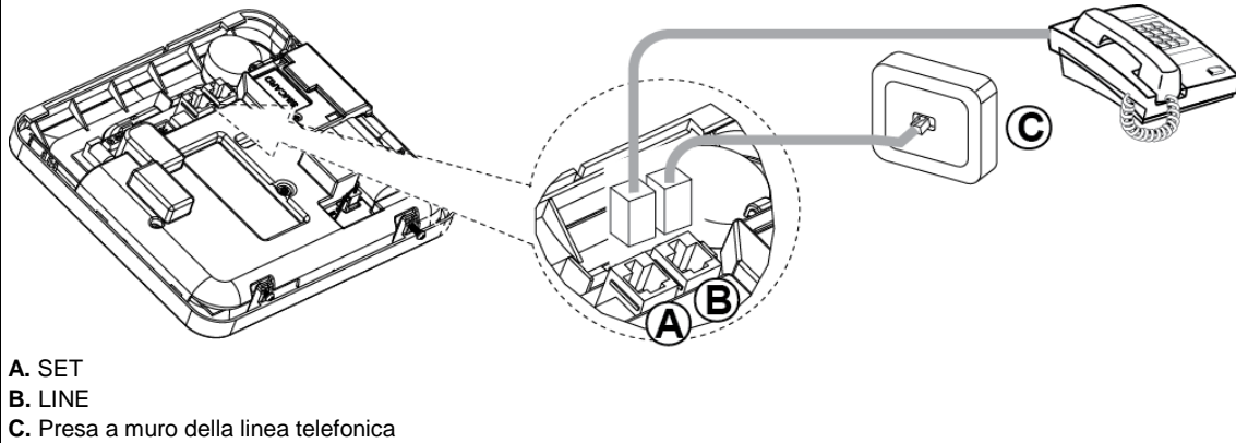
Figura 3.2 – Cablaggio del telefono
