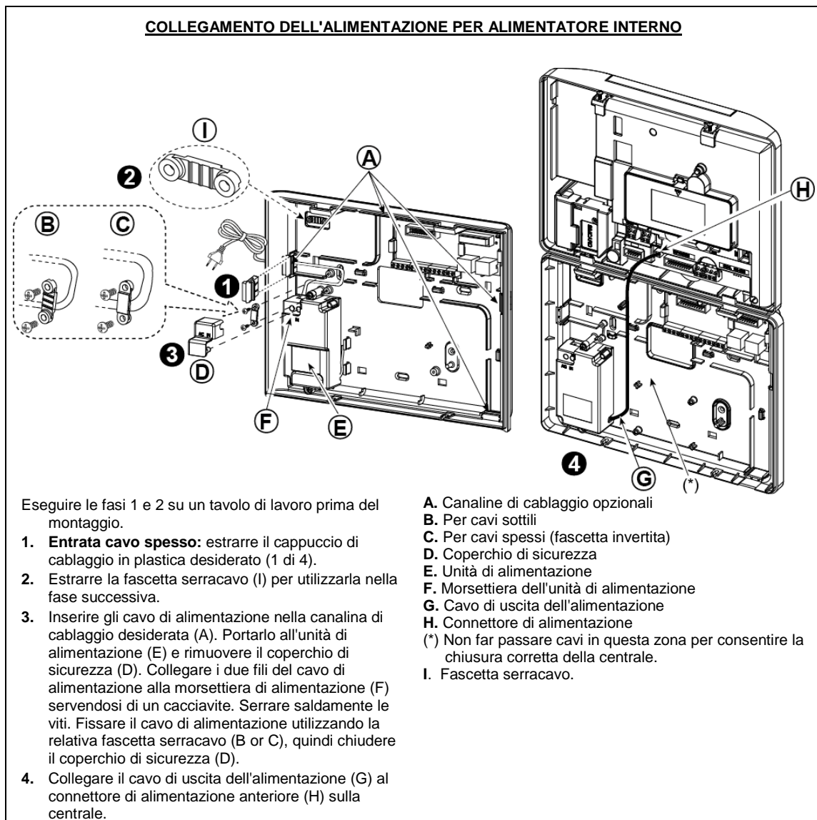
Figura 4.10a – Collegamento elettrico per alimentatore interno
