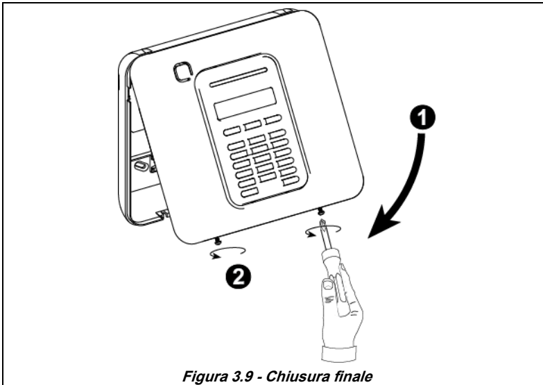
Figura 3.9 - Chiusura finale
