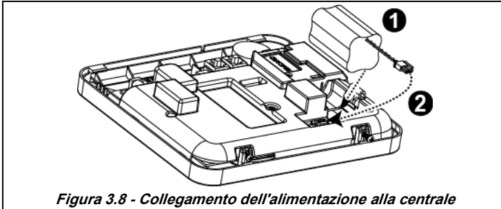
Figura 3.8 - Collegamento dell'alimentazione alla centrale
