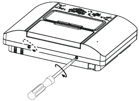
Figura 4.13 - Chiusura finale
