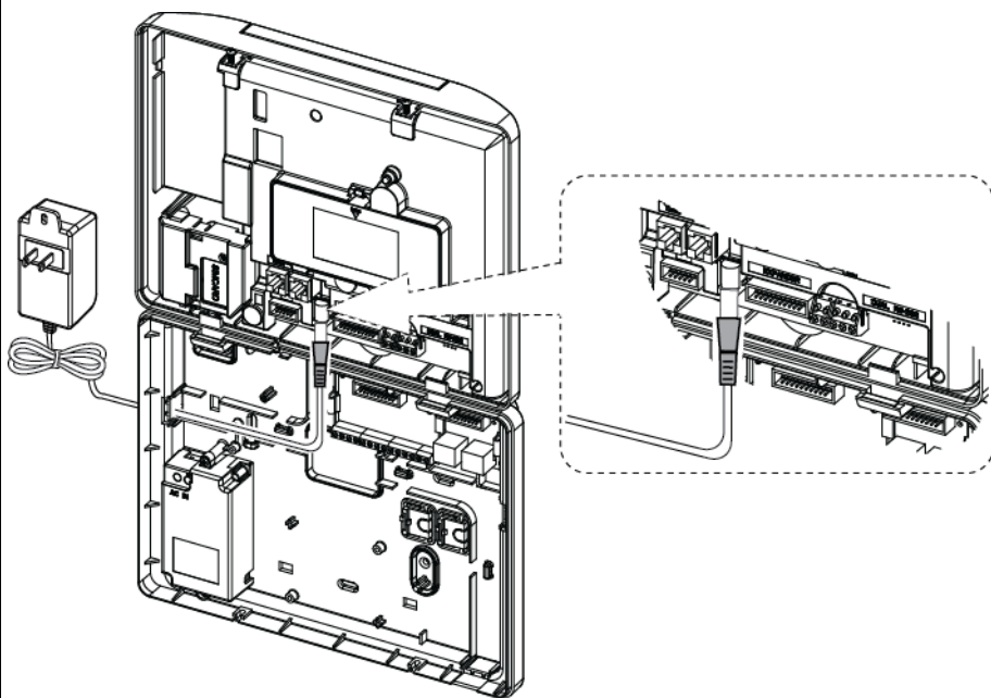
Figura 4.10b - Collegamento alimentatore esterno
