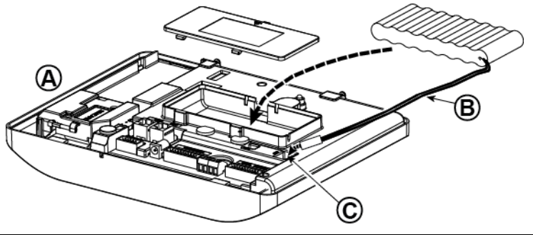
Figura 4.11 – Inserimento batterie
