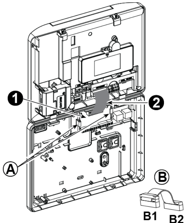
Figura 4.9a –Modulo Expander
