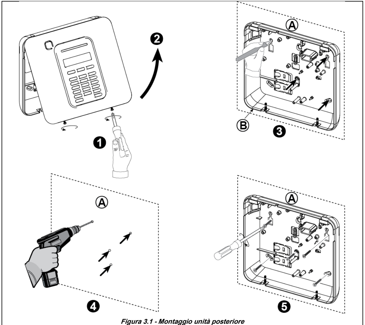
Figura 3.1 - Montaggio unità posteriore
