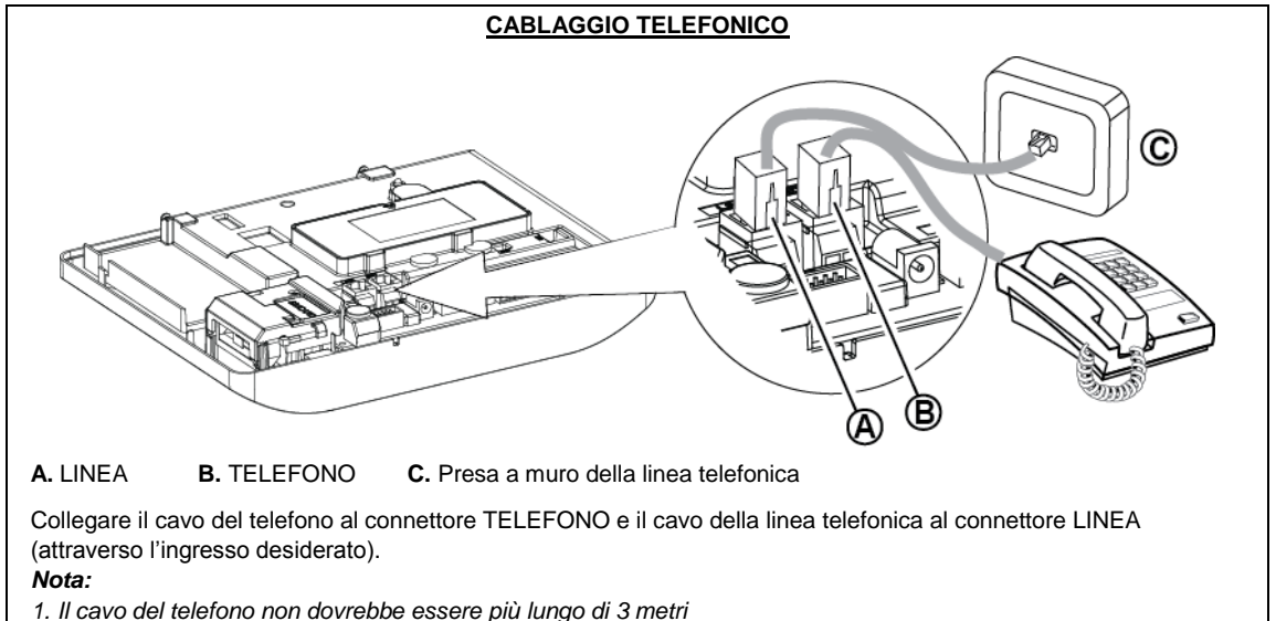
Figura 4.3a – Cablaggio telefono
