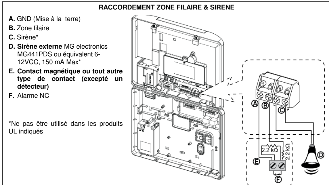
Schéma 4.4 – Raccordement zone filaire et sirène
