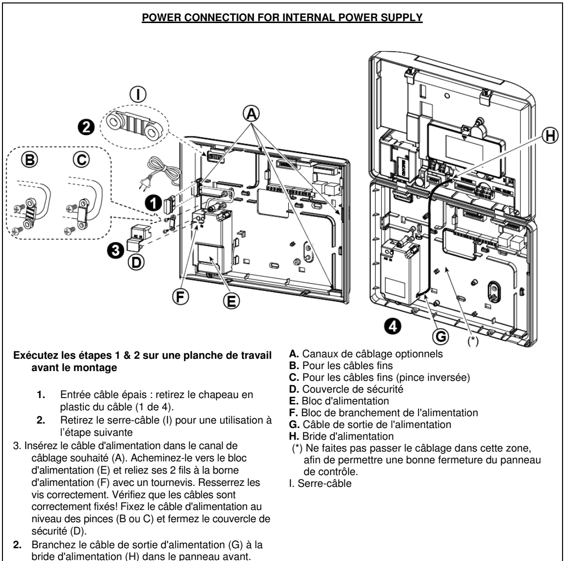
Schéma 4.10a – Raccord d'alimentation pour alimentation interne
