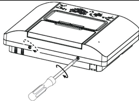
Schéma 4.14 - Fermeture finale
