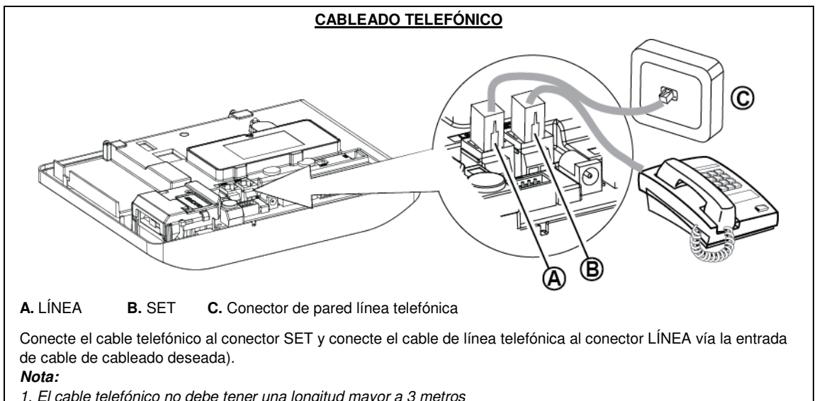
Figura 4.3a – Cableado Telefónico
