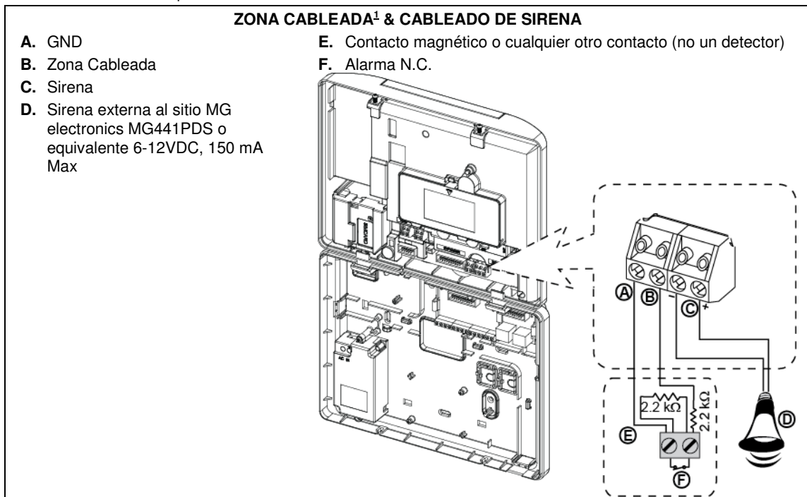
Figura 4.4 – Zona Cableada y Cableado de Sirena
