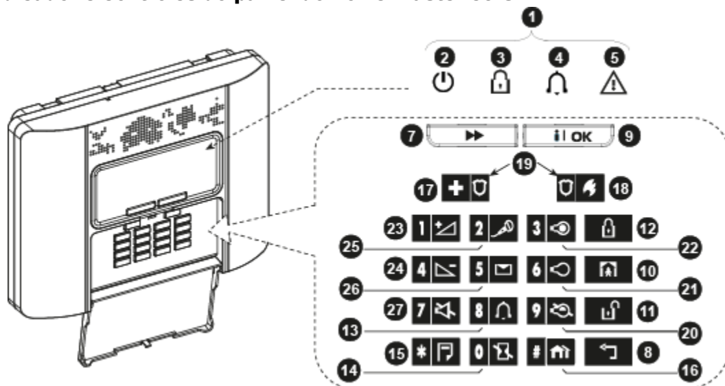
Figura 1b. Controles e indicadores do PowerMaster-30 G2
