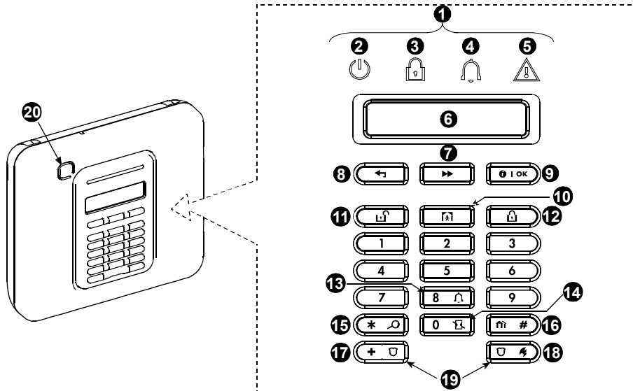
Figura 1a. Controles e indicadores do PowerMaster-10 G2
