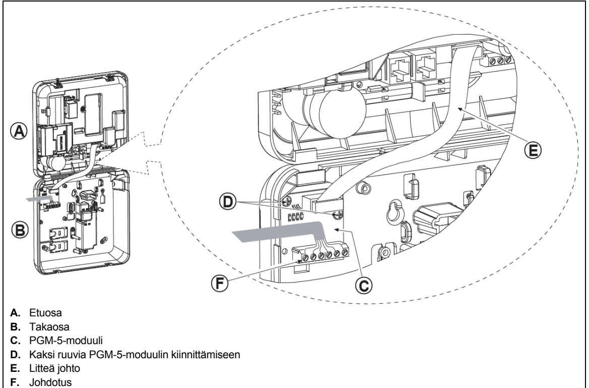
Kuva 3.5 – PGM-5-moduulin asennus
