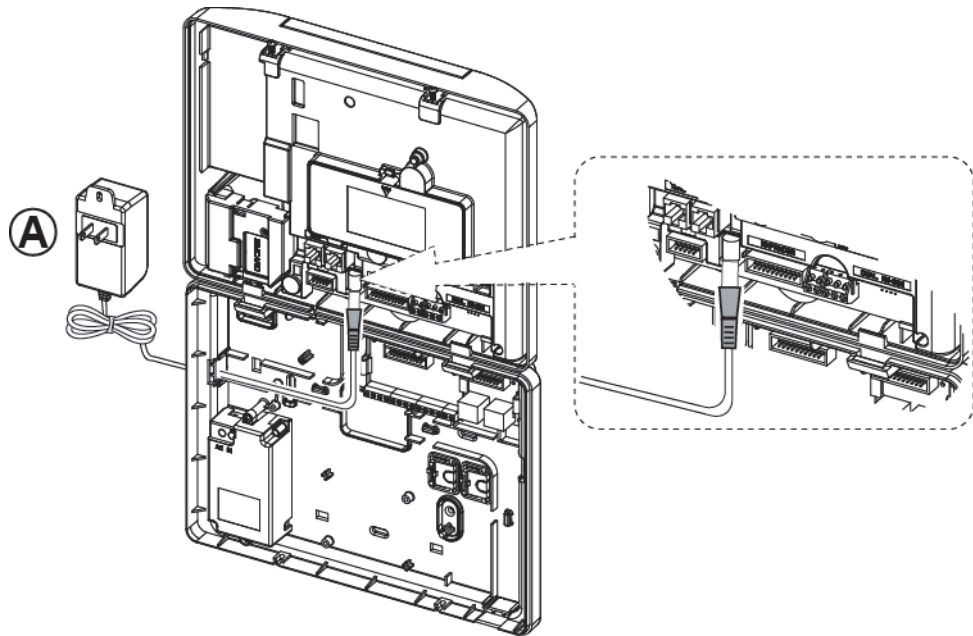
Kuva 4.10b. – Ulkoisen virtalähteen liitäntä
