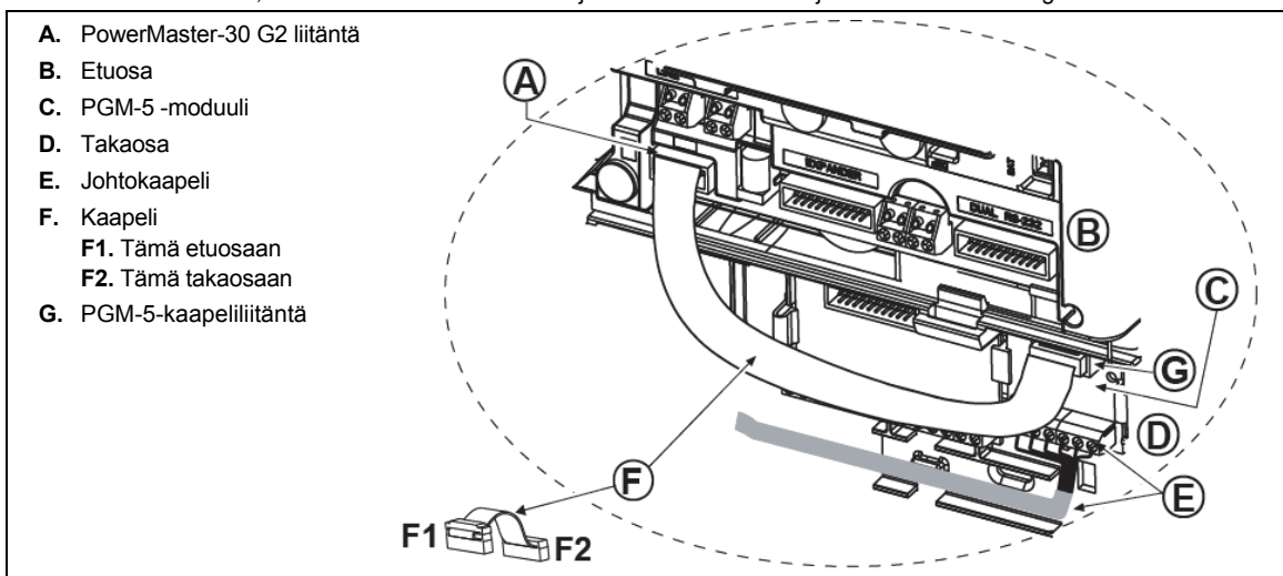
Kuva 4.8 – PGM-5-moduulin asennus
