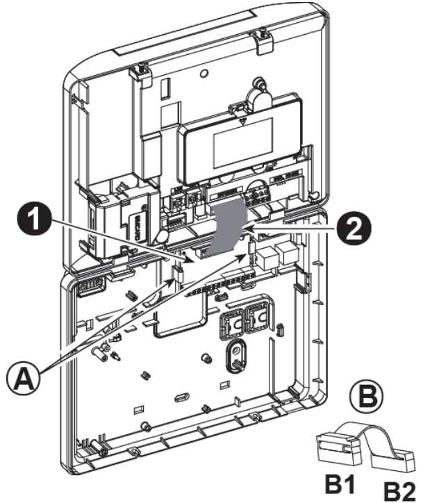
Kuva 4.9a – Laajennusmoduulin asennus
