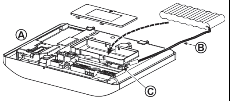
Kuva 4.11 – Patterien asentaminen
