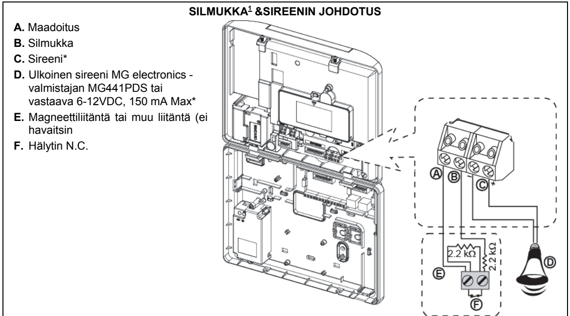
Kuva 4.4 – Silmukka- ja sireenijohdotus
