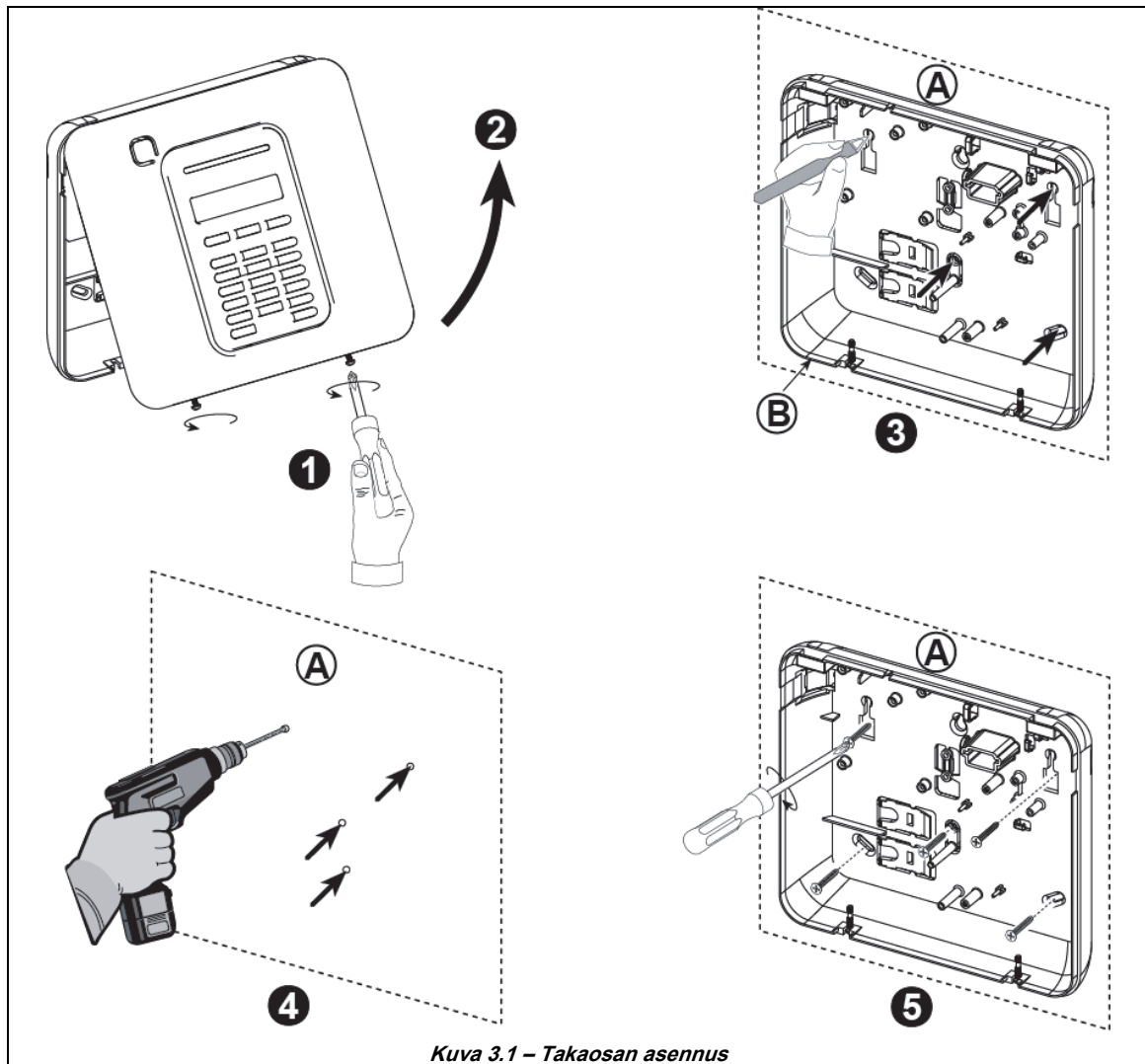
Kuva 3.1 – Takaosan asennus
