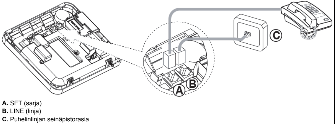
Kuva 3.2 – Puhelimen johdotus
