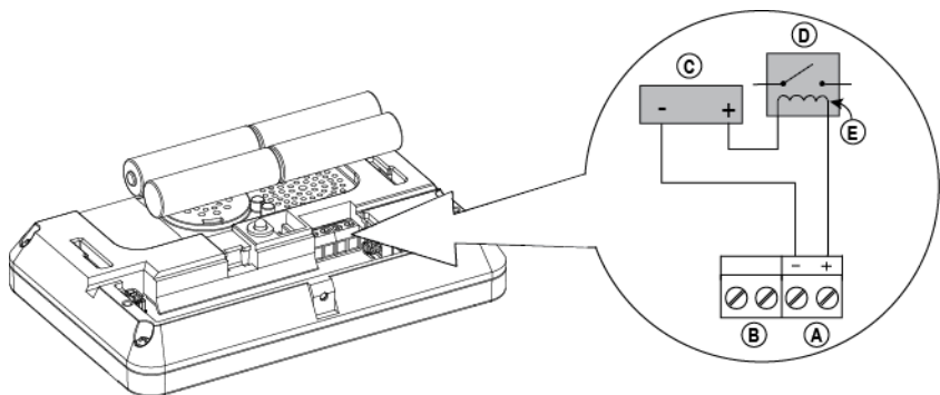
Figure 4 : connecteur externe
