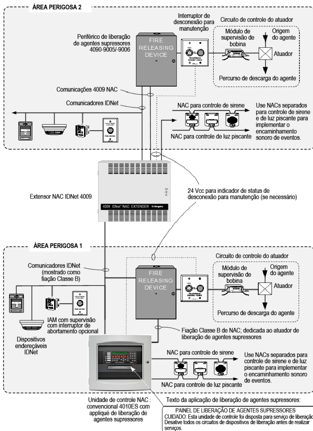
Figura 1: Referência de conexão de uma linha
