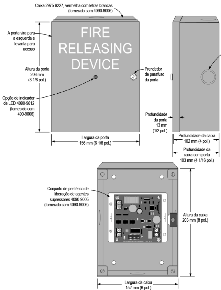
Figura 4: Diagrama de referência de instalação
