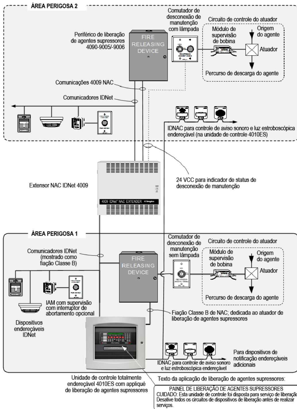
Figura 2: Referência de Conexão de Uma Linha
